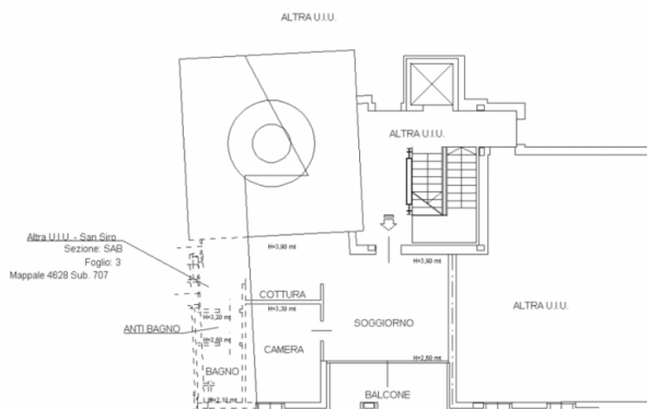
PIANTA PIANO PRIMO H = 2.70 Mt.
