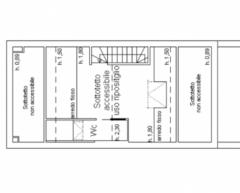
PIANO SECONDO. 2,70
