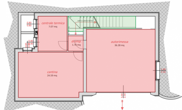
scala 1:100
