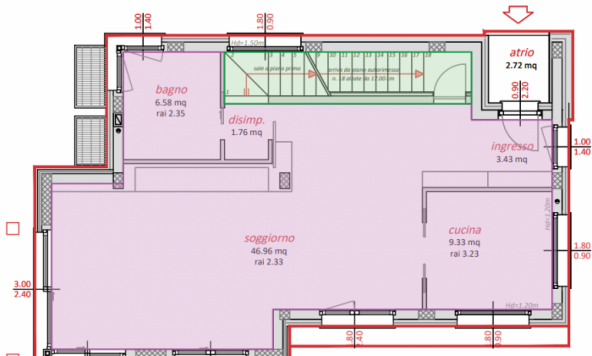
scala 1:100
