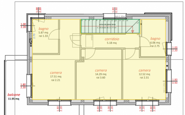
scala 1:100
