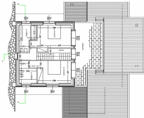
PIANTA PIANO PRIMO - 1. 100
