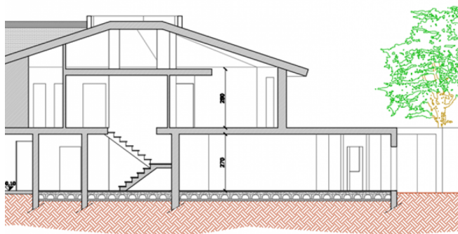
SEZIONE A - A
