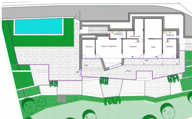
PIANTA SECONDO PIANO SOTTOSTRADA
