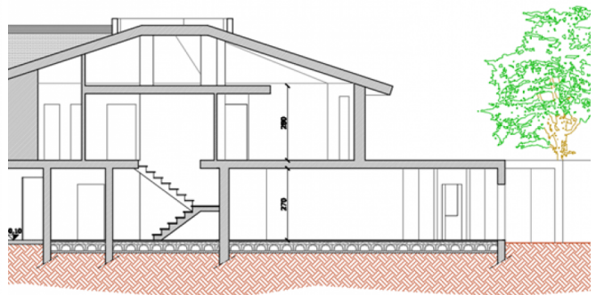
SEZIONE A - A
